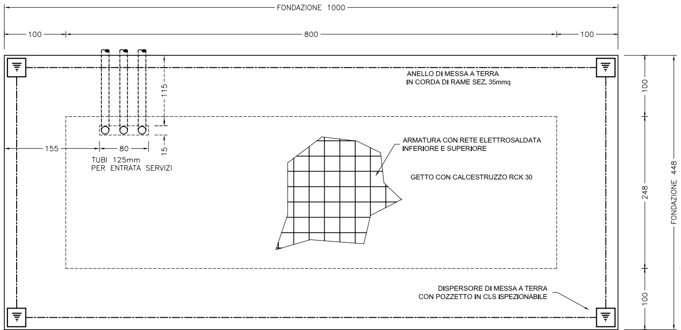
PIANTA FONDAZIONE
