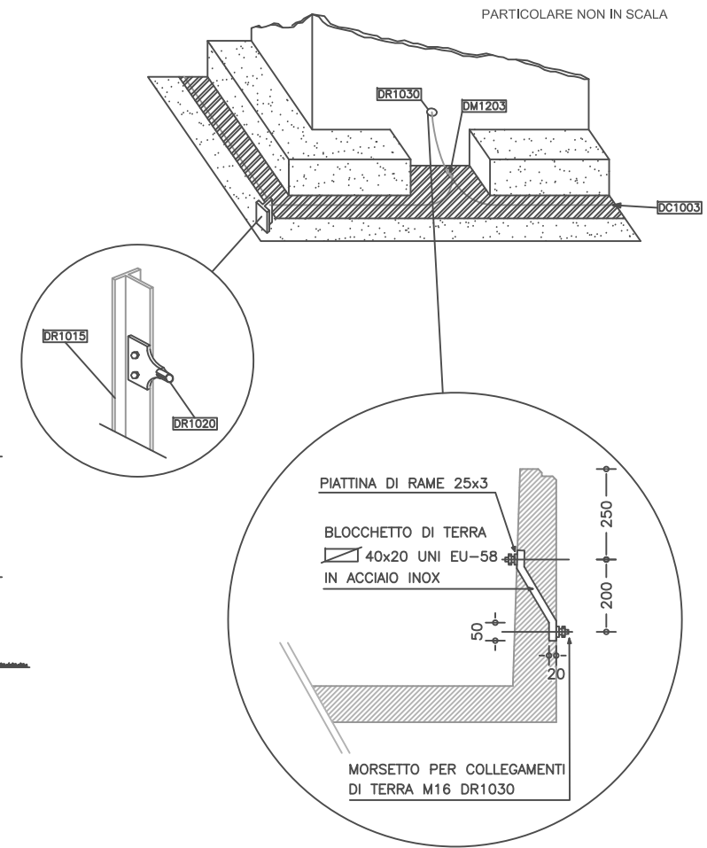
PARTICOLARE CONNETTORE INTERNO-ESTERNO RETE DI TERRA
