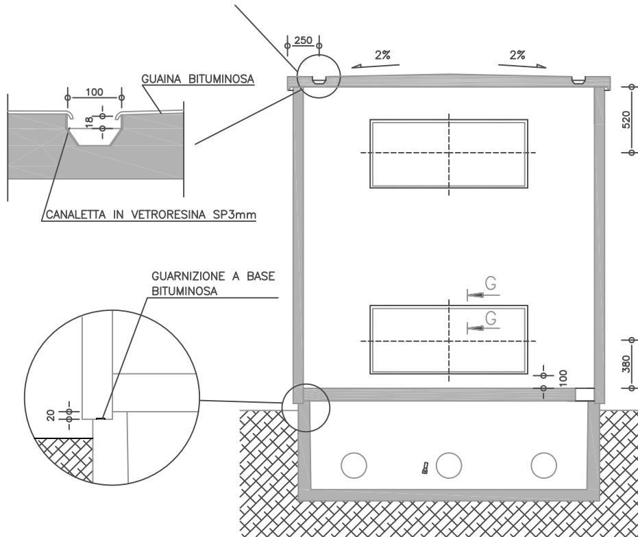
SEZIONE A-A
