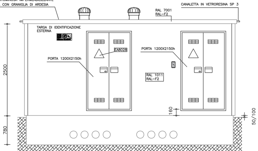
PROSPETTO FRONTALE
