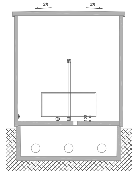
SEZIONE I-I
