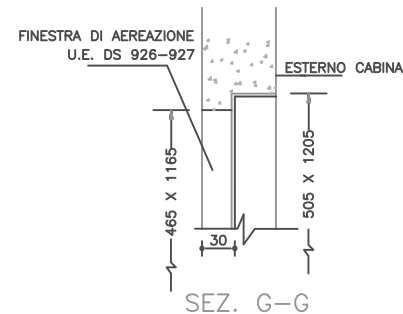
SEZ. G-G
