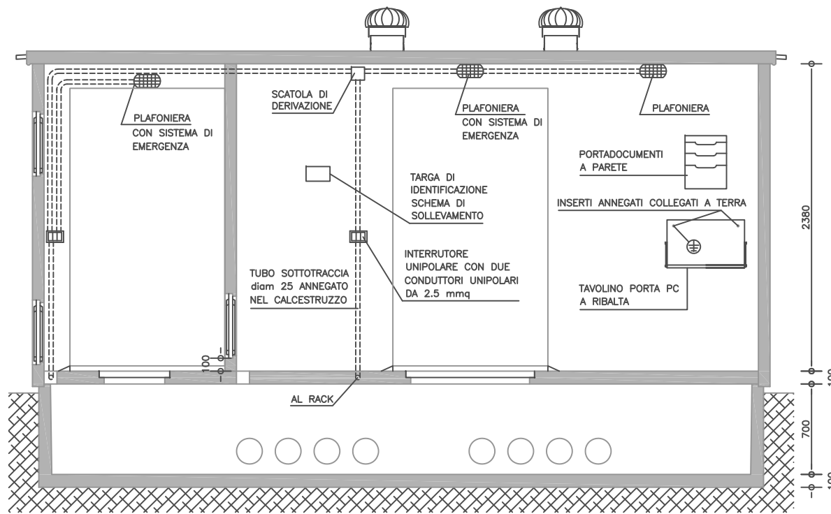
SEZIONE C-C
