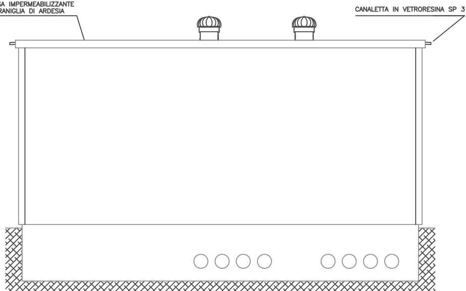
PROSPETTO RETRO
