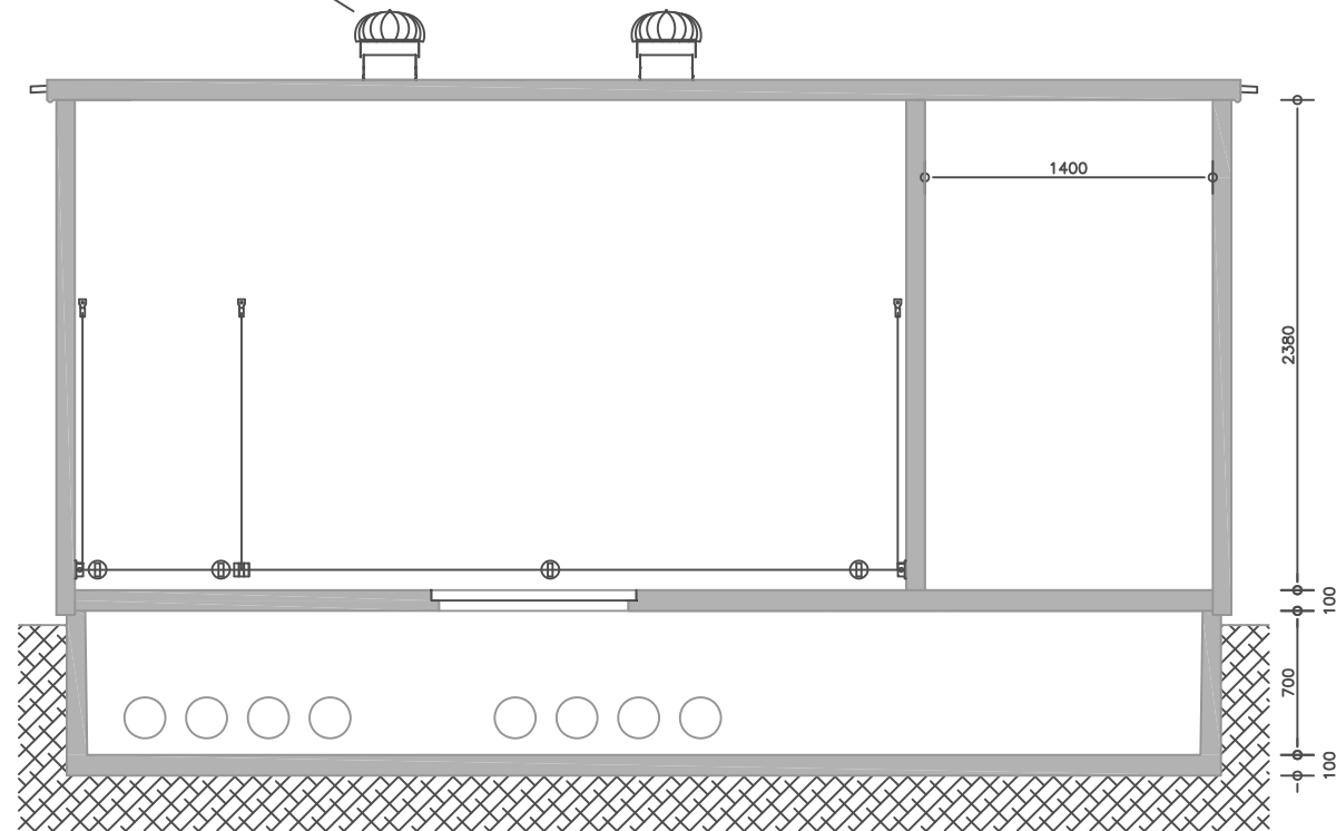
SEZIONE B-B
