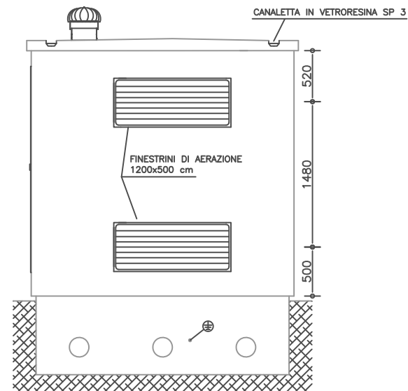
FIANCO DESTRO
