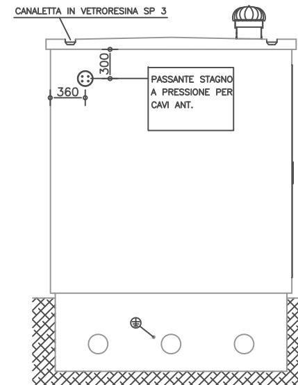
FIANCO SINISTRO
