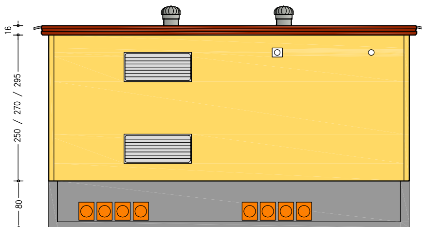
PROSPETTO SINISTRO
