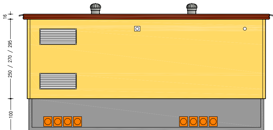
PROSPETTO SINISTRO
