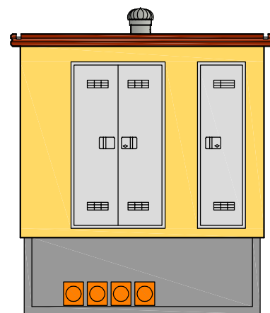
PROSPETTO FRONTALE
