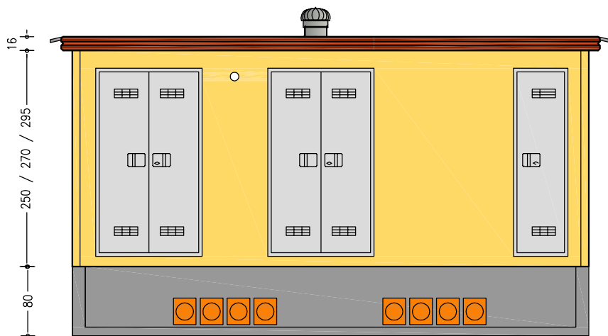
PROSPETTO FRONTALE
