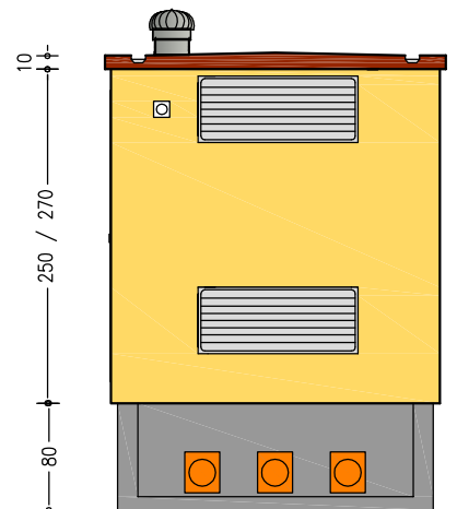
PROSPETTO DESTRO
