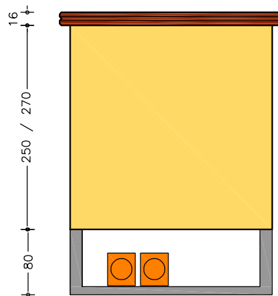
PROSPETTO SINISTRO
