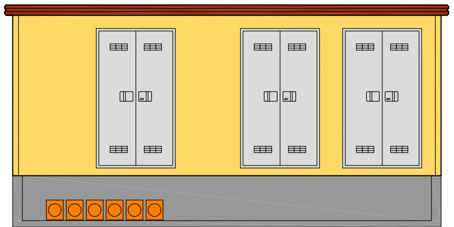
PROSPETTO FRONTALE
