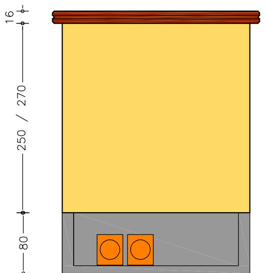
PROSPETTO SINISTRO
