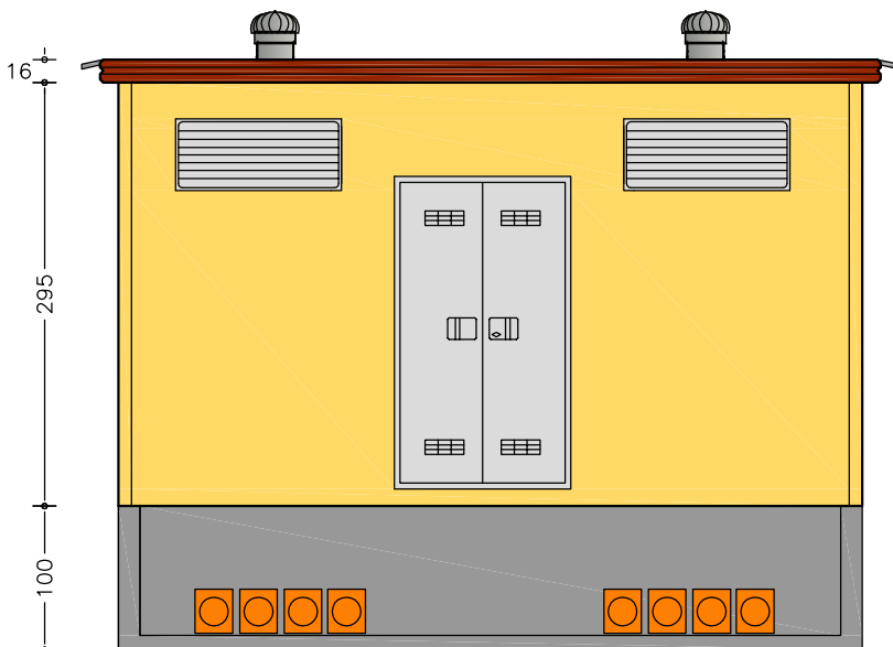
PROSPETTO FRONTALE
