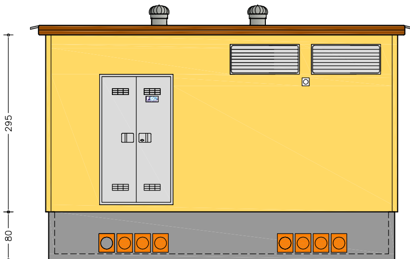
PROSPETTO FRONTALE
